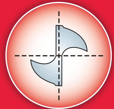
Klassische Spannute
